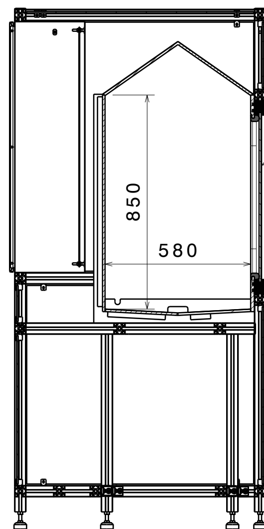
Schnitt A-A
