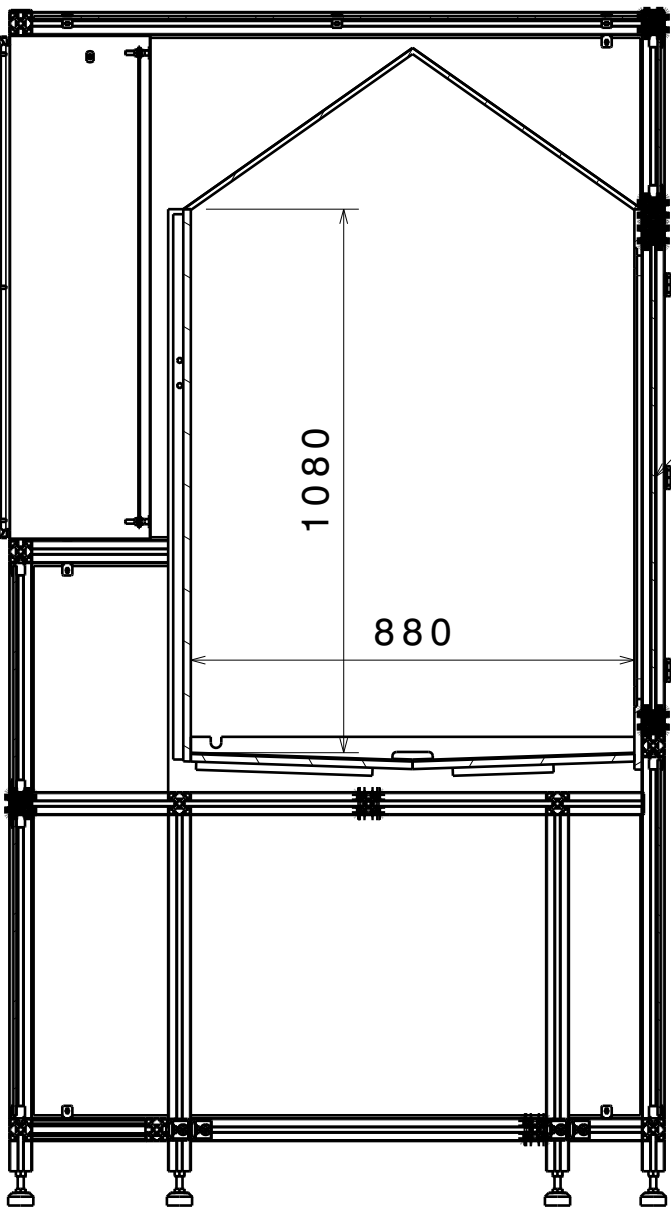
Schnitt A-A
